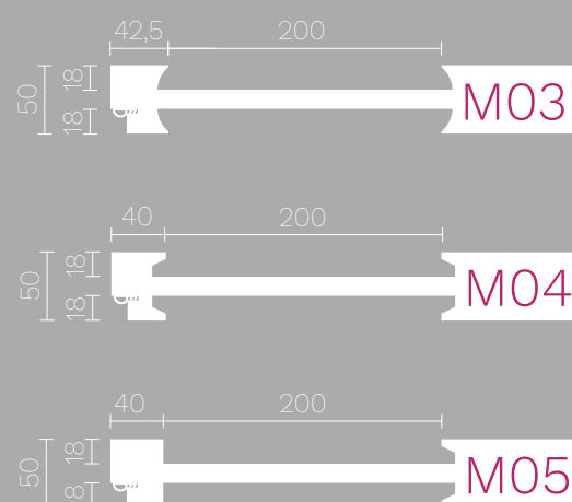
SEZIONI MANIGLIA SECTION OF BUILT-IN HANDLE
